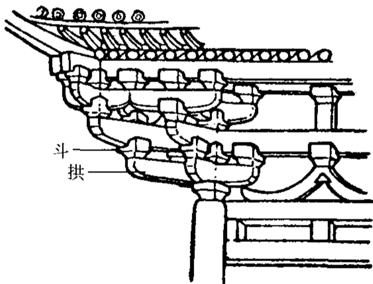
斗 拱
